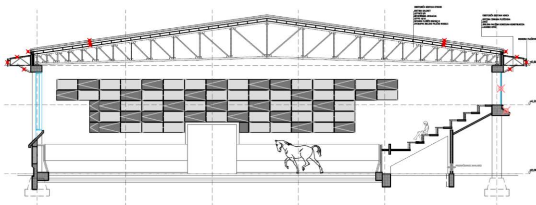
Slika 2: Prikaz objekta Velika jahalnica, iz katerega se odstranjuje strešno kritino, v prečnem prerezu. (Mašera mahnič arhitekti d.o.o.)
